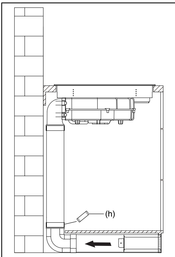
14. Fixieren Sie die Teile mit dem Klebeband.
