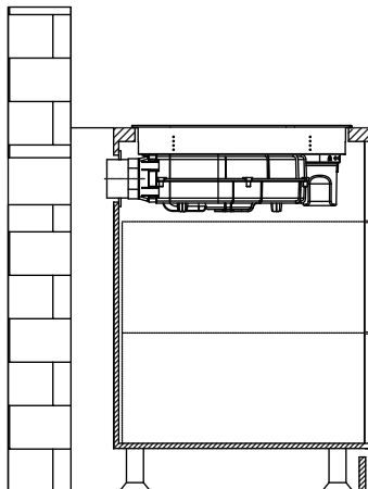
Recirculation A
