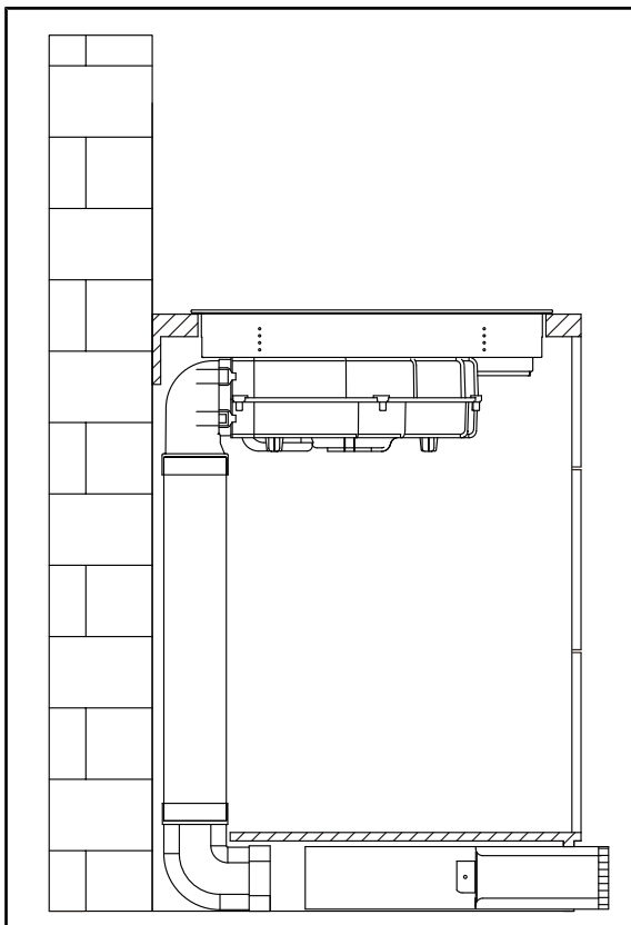
13. Installieren Sie den Umluft-Schrankadapter unter dem Einbauschränk.
