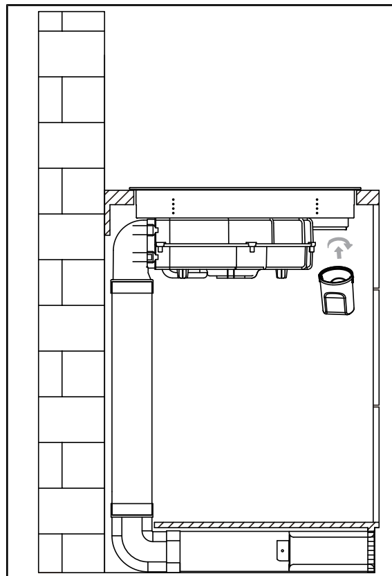
15. Befestigen Sie den Wasserauffangbehälter (a).
