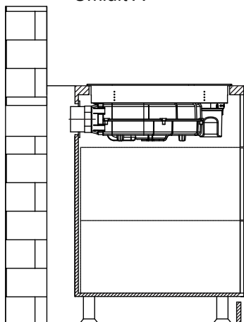
Umluft A
