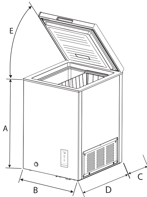
HGT8550EE
